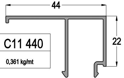
CAM KALINLIĞINA GÖRE CAM ÇİTASI SEÇİM TABLOSU ASİMETRİK CAM TABLOSU Glazing Bead Selection Table according to the Glass Thickness Asymmetric Glass List
