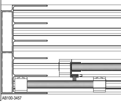
AB100 - SÜRME CAM BALKON SİSTEMİ Glass Slide System
