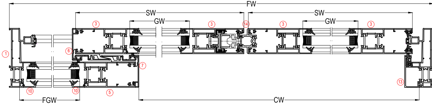
CAM KESİM ÖLÇÜLERİ / GLASS CUTTING SIZES
